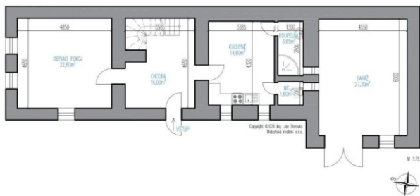
CHALUPA KLÁŽARY – PŘÍZEMÍ
