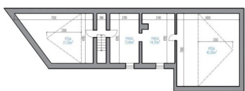
Podzemní plán Dlešní Bukovsko - 2.NP
