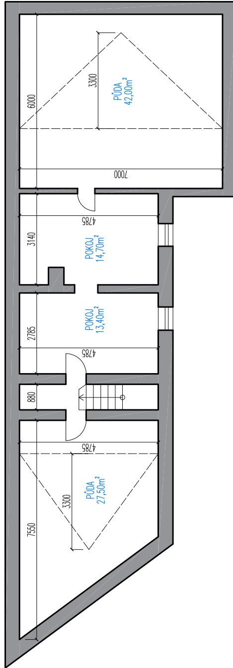
Rodinný dům Dolní Bukovsko – 2.NP
